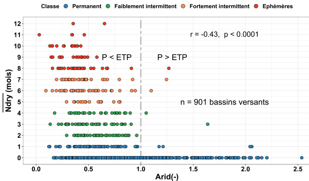
Figure III-16 : Relation linéaire simple entre la moyenne du nombre de mois secs et l'indice d'aridité (Arid) pour les 901 stations de calibration.
