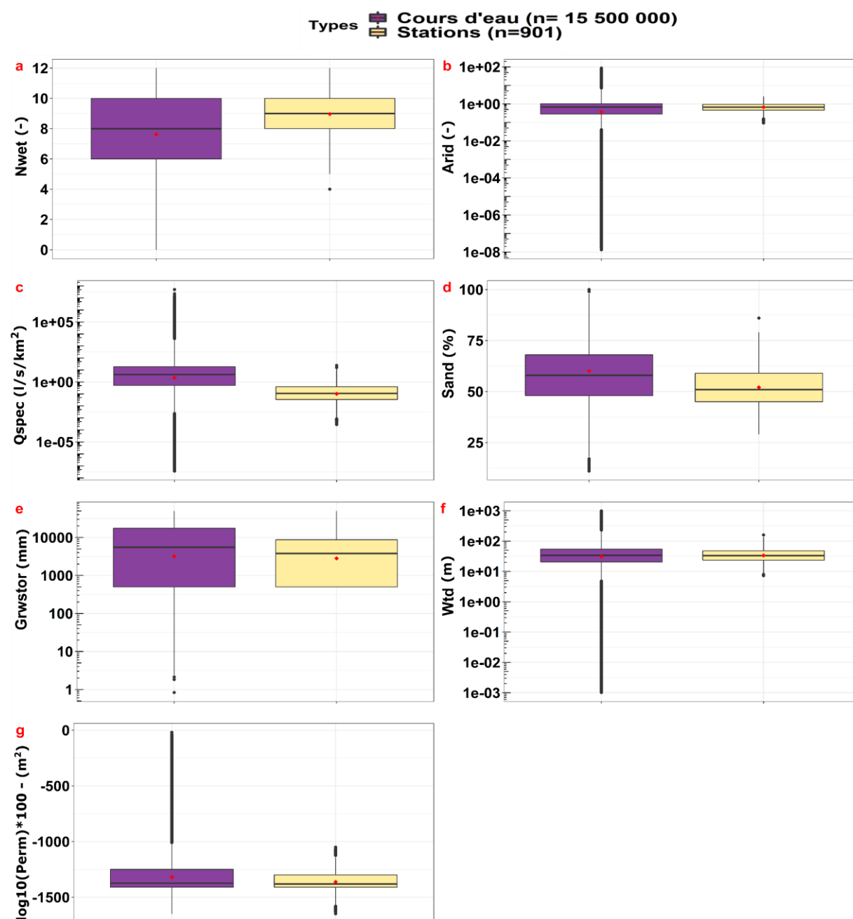
Figure III-18 : Distribution des variables hydro-environnementales pour 15 500 000 bassins versants amont associés aux tronçons de rivières (couleur violette) et 901 bassins versants amont associés aux stations de jaugeage utilisés en calibration des modèles. a) Nwet, b) Arid, c) Qspec, d) Sand, e) Grwstor, f) Wtd, g) Perm. Les noms complets des variables sont définis dans le Tableau III-2 .
