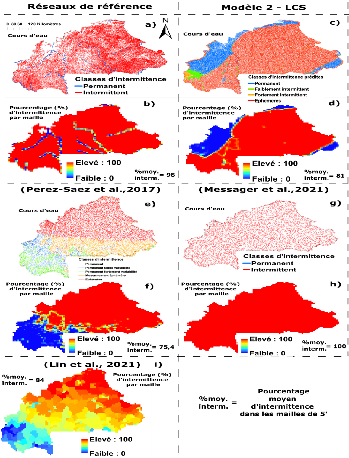
Figure II-A-18 : Comparaison de la distribution spatiale de l'intermittence prédite par M2-LCS-BF et les études (Lin et al., 2021 ; Messenger et al., 2021 ; Perez-Saez et al., 2017) à la carte nationale de l'intermittence (IGB-BNDT) du Burkina Faso.
