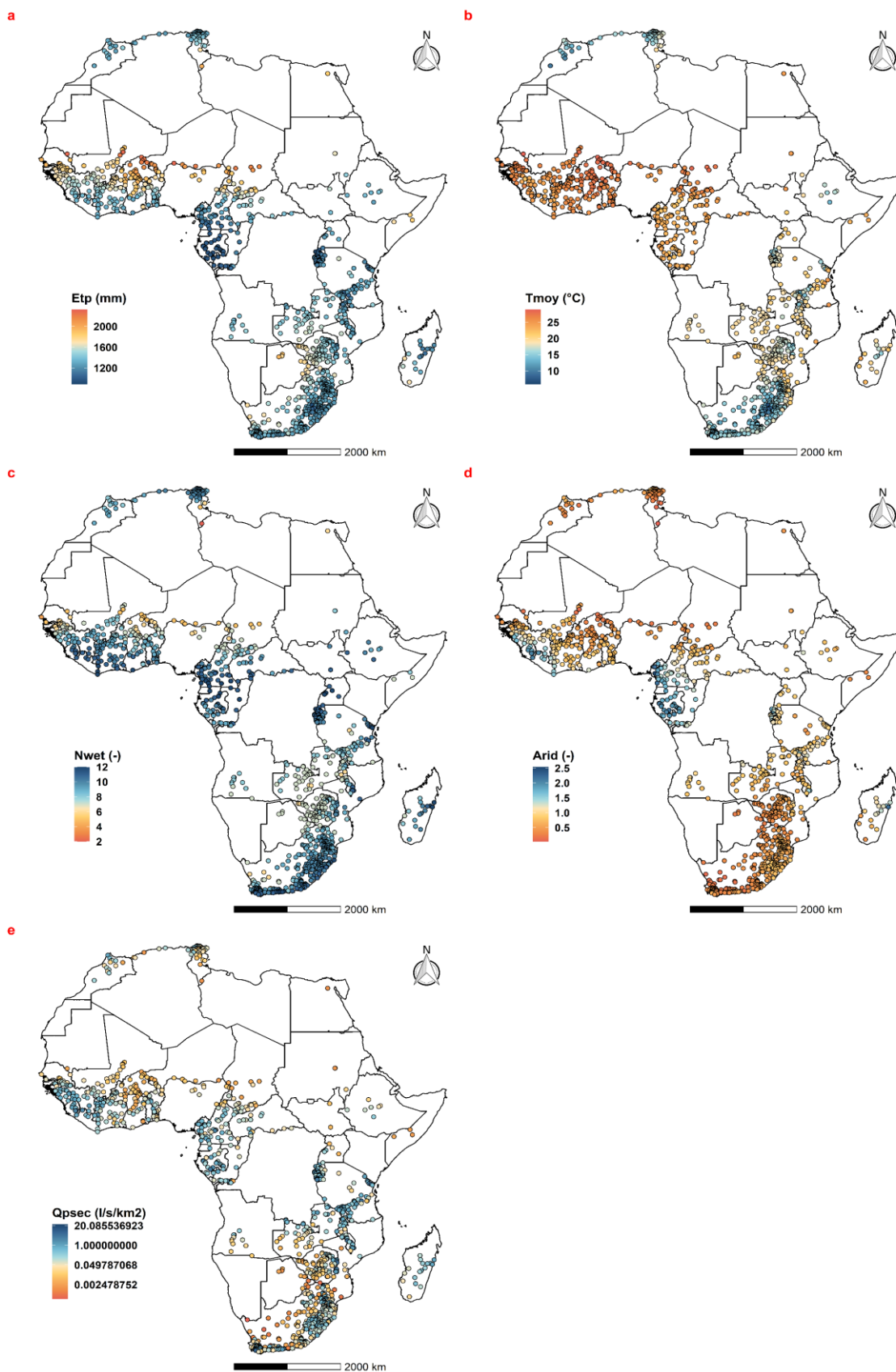
Figure A3-2 : Caractéristiques hydro-climatiques des 1125 bassins versants en Afrique. Les points représentent les exutoires des bassins versants.
