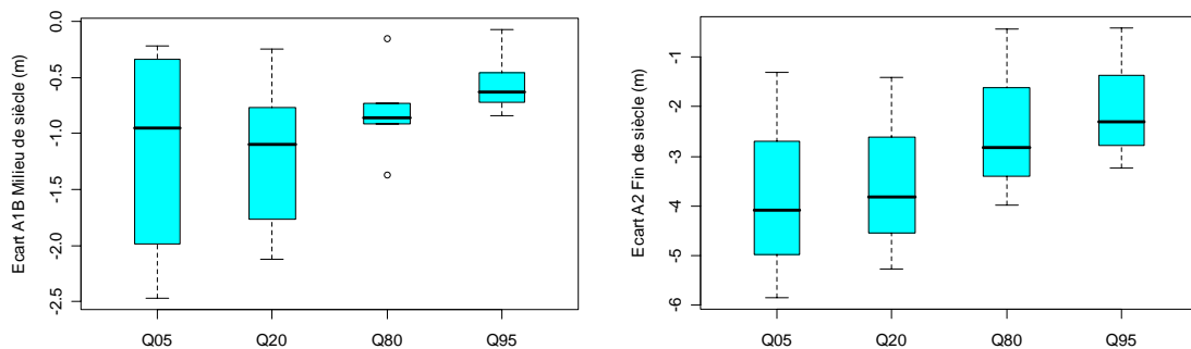
Figure 17 - Evolution des quantiles de niveaux piézométriques dans le bassin de la Somme selon GARDENIA. Les écarts sont évalués par rapport aux résultats sous scénarios désagrégés temps présent. Les scénarios A1B fin de siècle n'ont pas été simulés par ce modèle.
