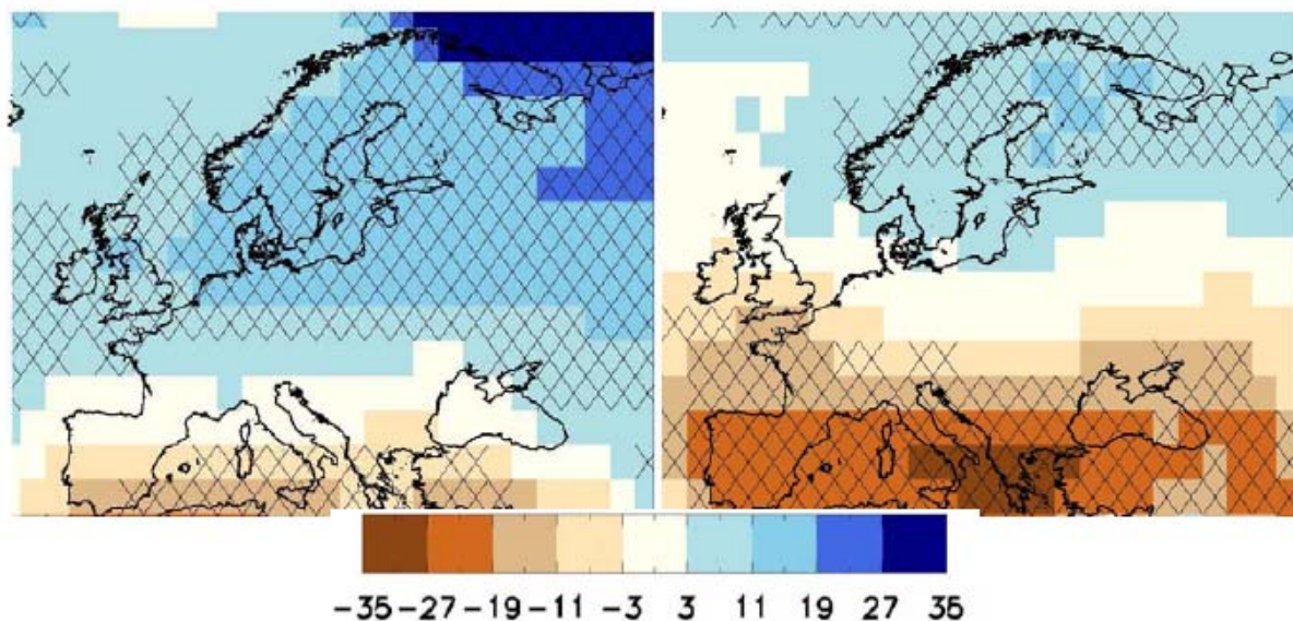
Figure 2 – Europe : changement relatif (par rapport à la période 1971-2000) des précipitations hivernales (à gauche) et estivales (à droite) simulées par le multi-modèle CMIP3 pour la période 2046-2065 et le scénario d'émissions SRES A1B. Les croix indiquent les zones où au moins 85% des signes des réponses des différents modèles sont en accord (source : Boé, 2007).
