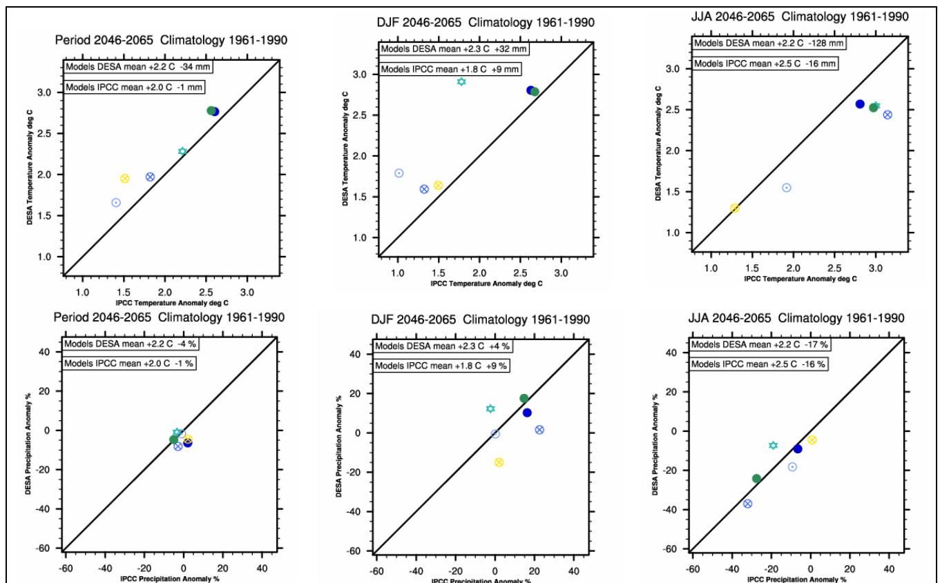
Figure 4 - Comparaison des changements des températures (en haut) et précipitations (en bas) simulés entre les périodes 2046-2065 et 1970-1999 pour le scénario SRES-A1B selon les 6 modèles du GIEC choisis pour le volet V2 : changements directement simulés par les modèles de climat en abscisse vs changements après désagrégation par la méthode RT en ordonnée. De gauche à droite la moyenne annuelle, la saison hivernale (DJF) et estivale (JJA).
